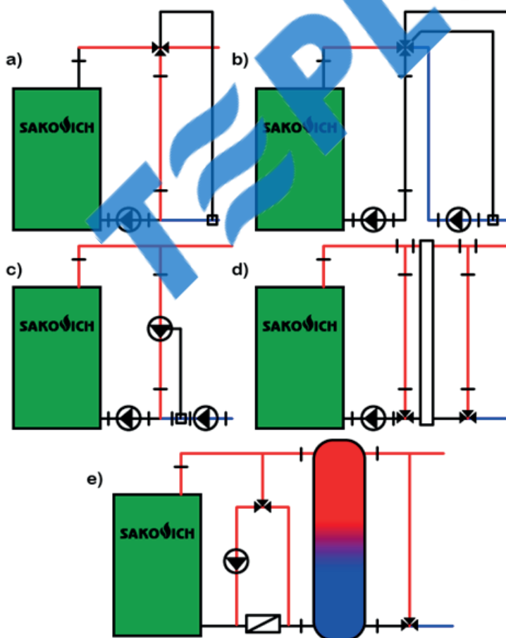
Рис 3. Рекомендуемые схемы соединения котла с системой отопления: а) с трехходовым клапаном; б) с четырех ходовым клапаном; в) с циркуляционным насосом; г) с гидравлической муфтой; д) с буферной ёмкостью.
