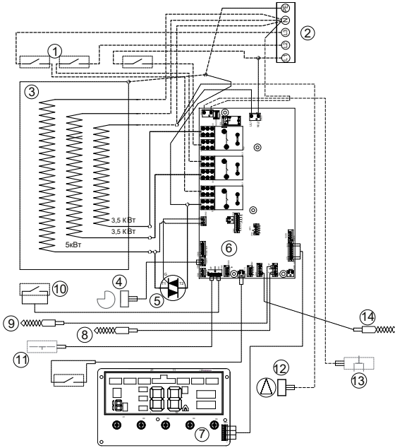
Схема подключений на плате управления
