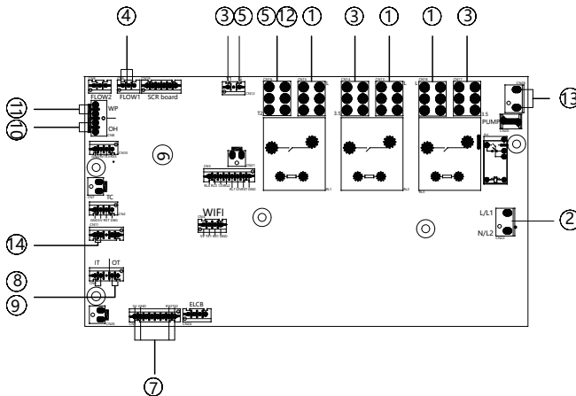
Схема подключений на плате управления
