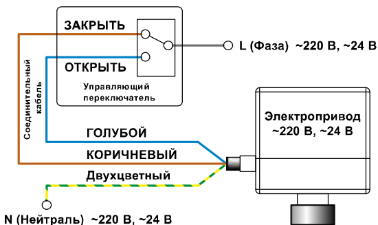
Рис. 1. Схема подключения и управления краном шаровым с электроприводом GL с напряжением питания 220 В ~50 Гц, 24 В ~50 Гц.
