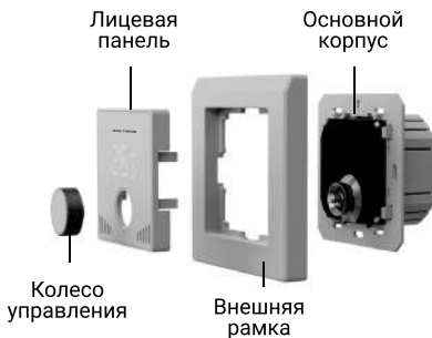
Рис. 3. Устройство терморегулятора
