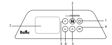
Рис. 2 Панель управления
