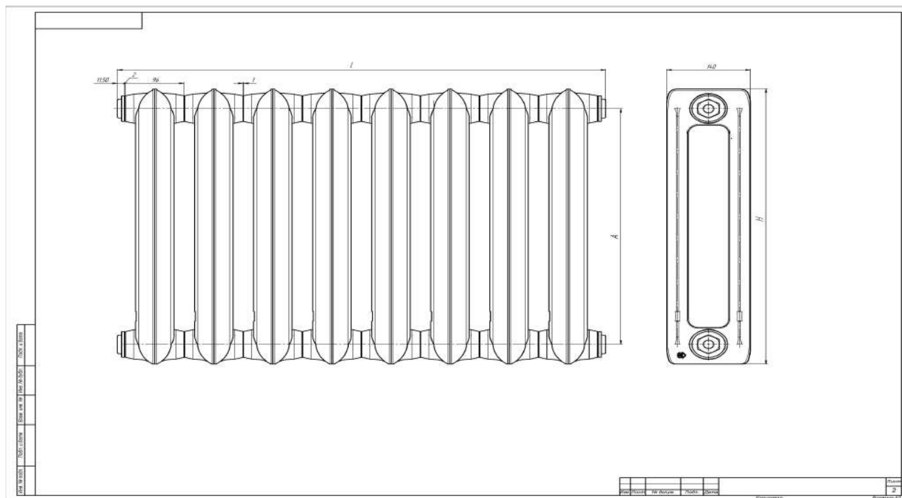
Рисунок 1 – Радиатор отопительный МС-140М4 500-1,2
