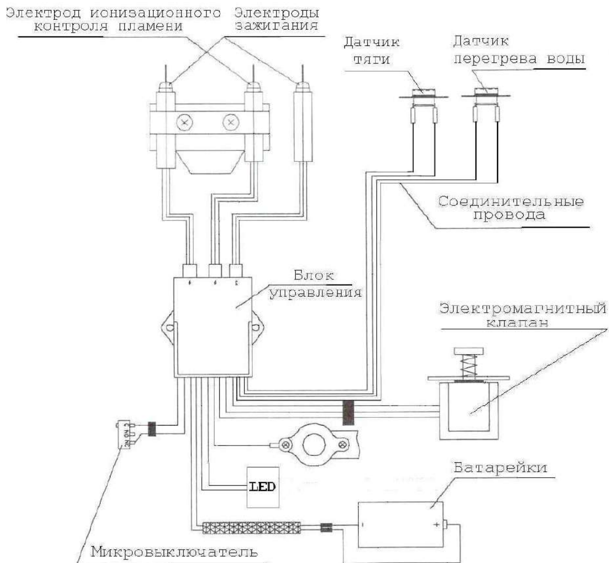
Рис. 2. Схема электрическая
